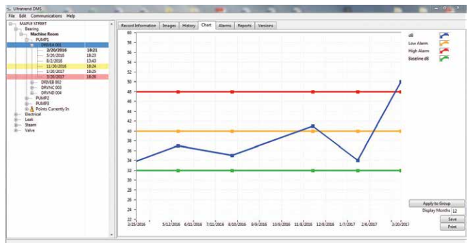
ULTRATREND DMS™ - Data İşleme Programı (Chart ekran görüntüsü)
