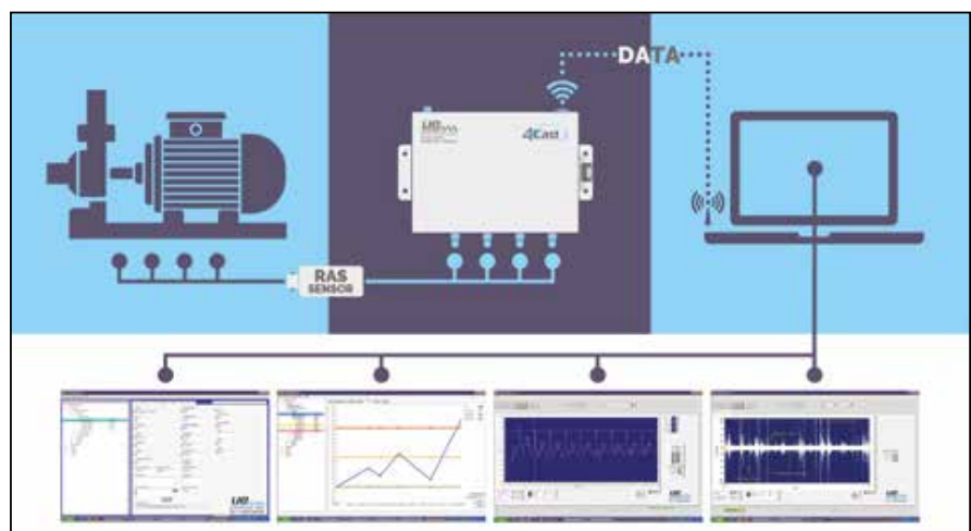
Schéma de principe : surveillance ultrasonore de machine tournante
